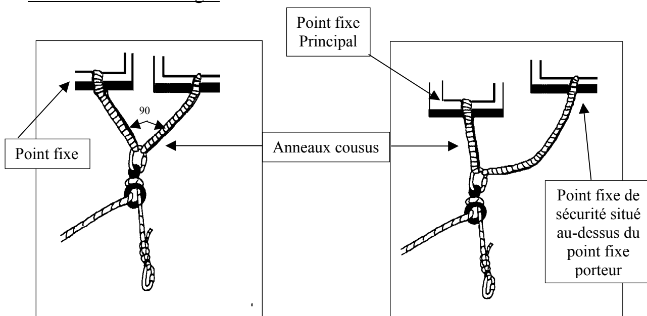
Répartition de la charge sur 2 points fixes
